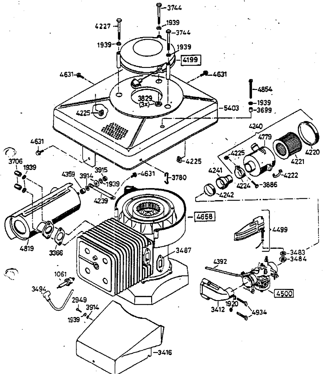
4657 Antriebsblock (mit Radantrieb) driving unit (wheel drive) moteur complet (autotracté)
